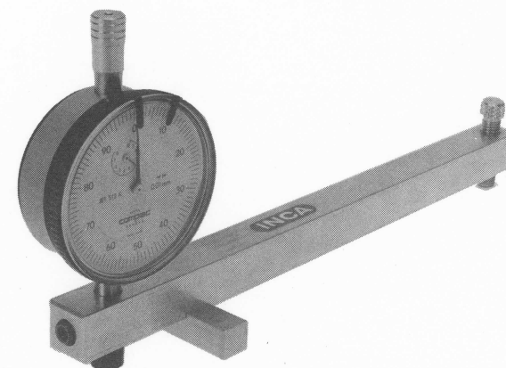
INCA-Einstellvorrichtung für Hobelmesser 348.196.03 Dispositif à régler les couteaux INCA INCA-Adjusting Device for Cutters
